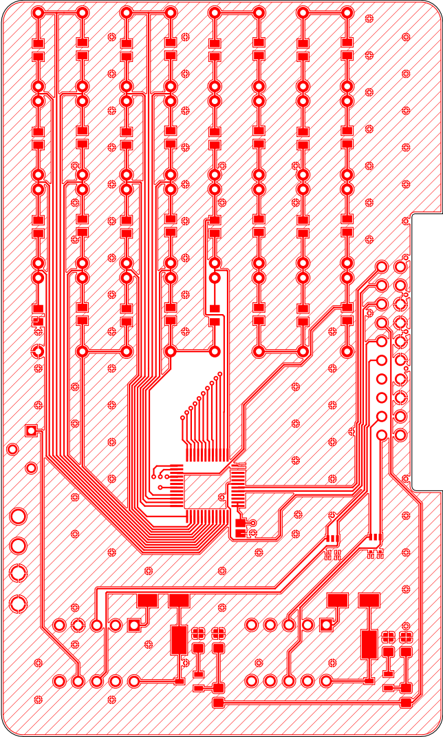
Top Layer (Scale 2:1)
