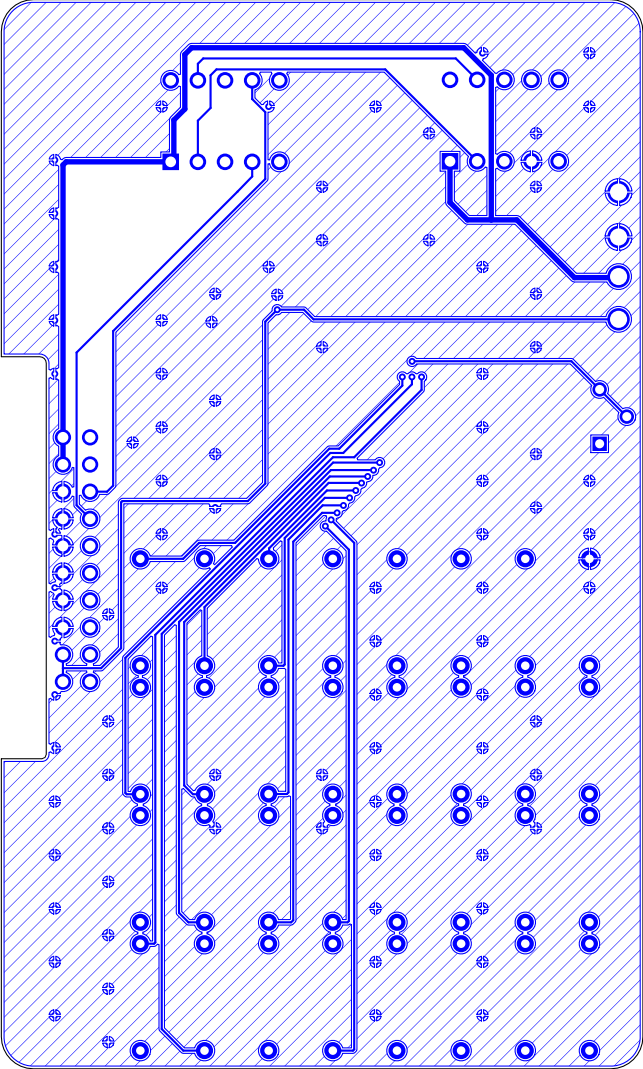
Bottom Layer (Scale 2:1)
